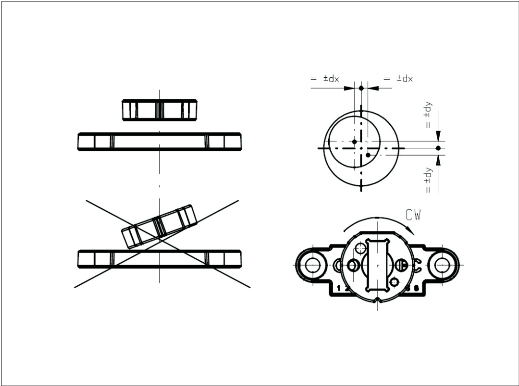
Vert-X 05E6 安装信息
